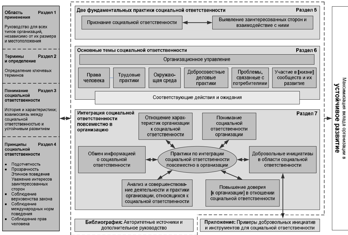
Рисунок 1 — Схема ИСО 26000
